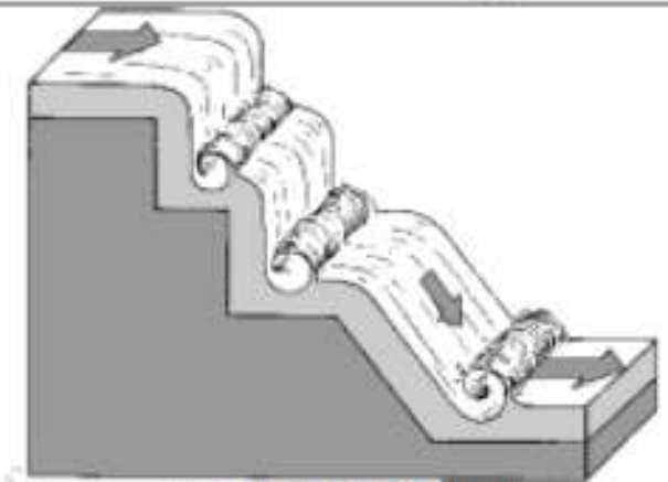
Ступенчатый слив.
